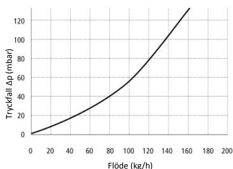
Tryckfallsdiagram
